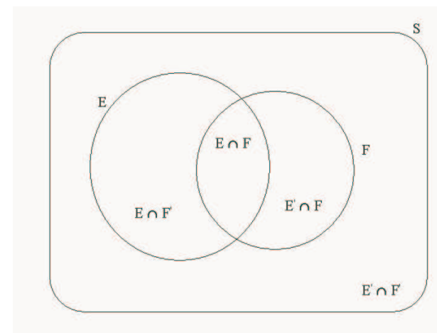
Venn Diagram
